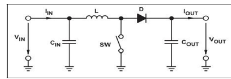
Gambar 1. Konfigurasi dasar boost converter Sumber : google.com
