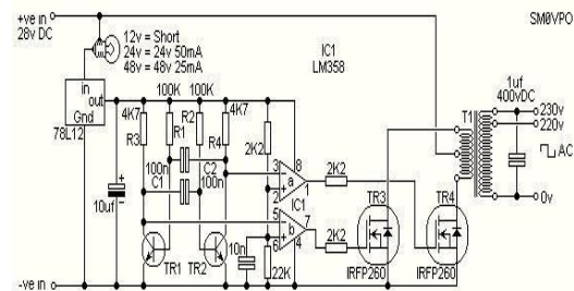
Gambar 2. Boost converter konversi energi hingga 12 V Sumber : google.com
