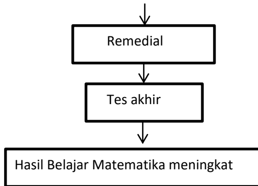
Gambar 2.1 Kerangka Pikir
